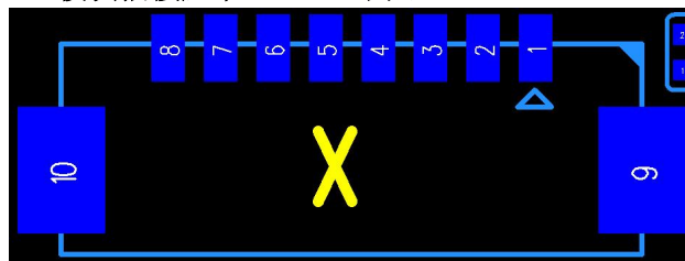
X 区：8 PIN DAB 模块插接座子 1.25mm 间距。
