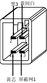
C 马自达4PIN母头4
