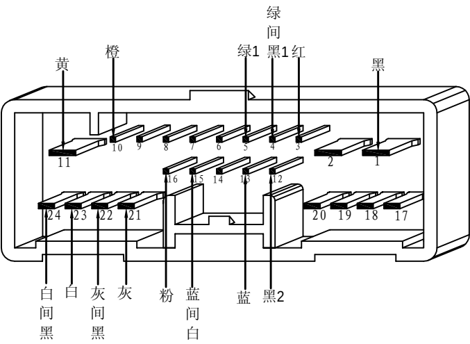
A 马自达24PIN大母头
