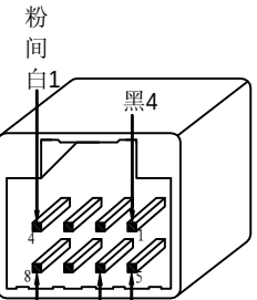
B 马自达8PIN母头
