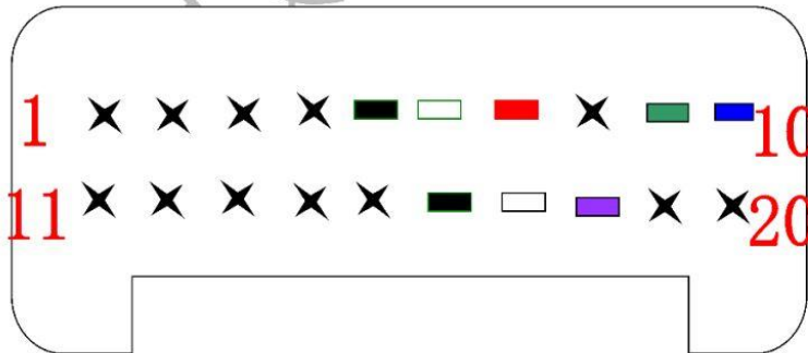
方控座
