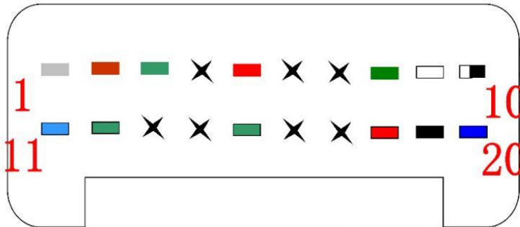
电源座
