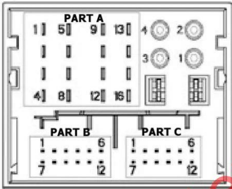
尾线端子 1(PartA)
