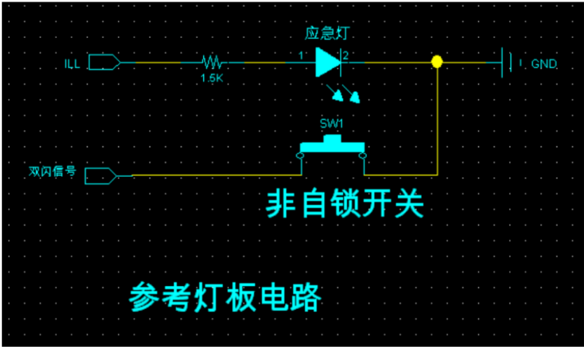
附 15 款锐界改装双闪按键灯板参考电路
